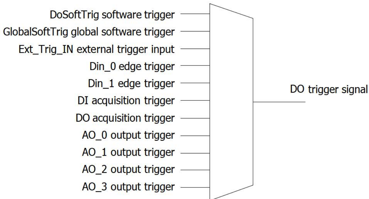
DO trigger options
