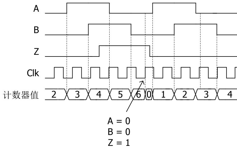
图 7.21 通道 Z 复位示例
