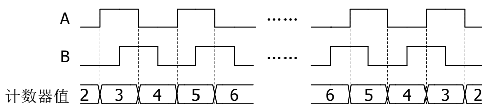
图 7.18 正交编码器 X2 编码计数方式
