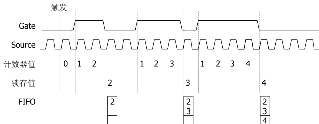
图 7.6 隐式缓冲脉宽采集示例
