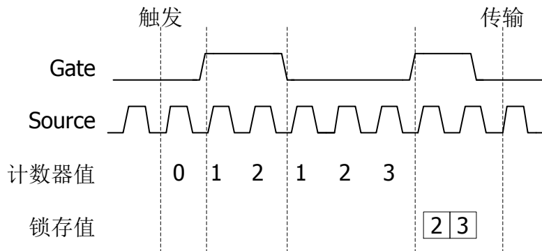
图 7.7 软件控制单点测量的示例
