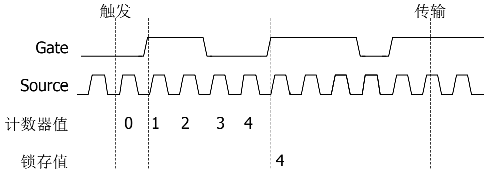
图 7.14 软件控制单点测量示例
