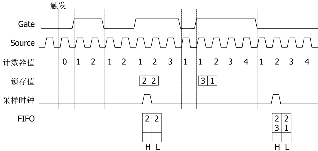
图 7.8 采样时钟定时连续采集示例
