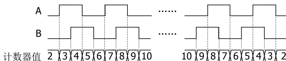
图 7.20 正交编码器 X4 编码计数方式
