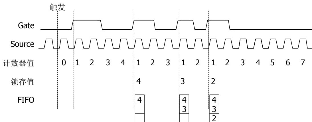
图 7.16 隐式缓冲频率测量示例
