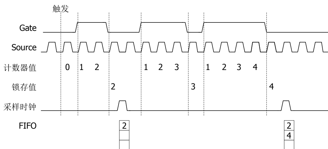
图 7.5 采样时钟定时连续采集示例
