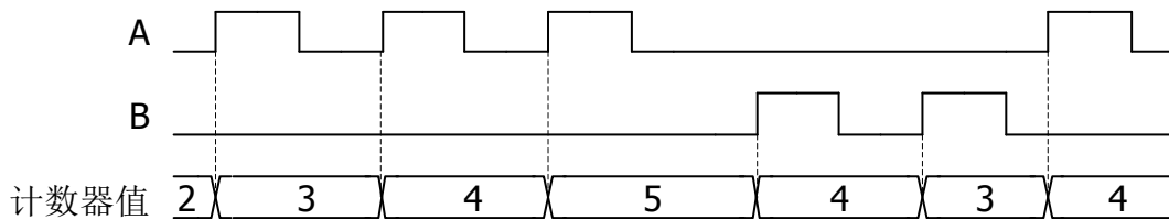
图 7.22 双脉冲编码器测量示例
