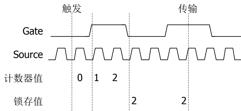
图 7.4 软件控制单点测量的示例
