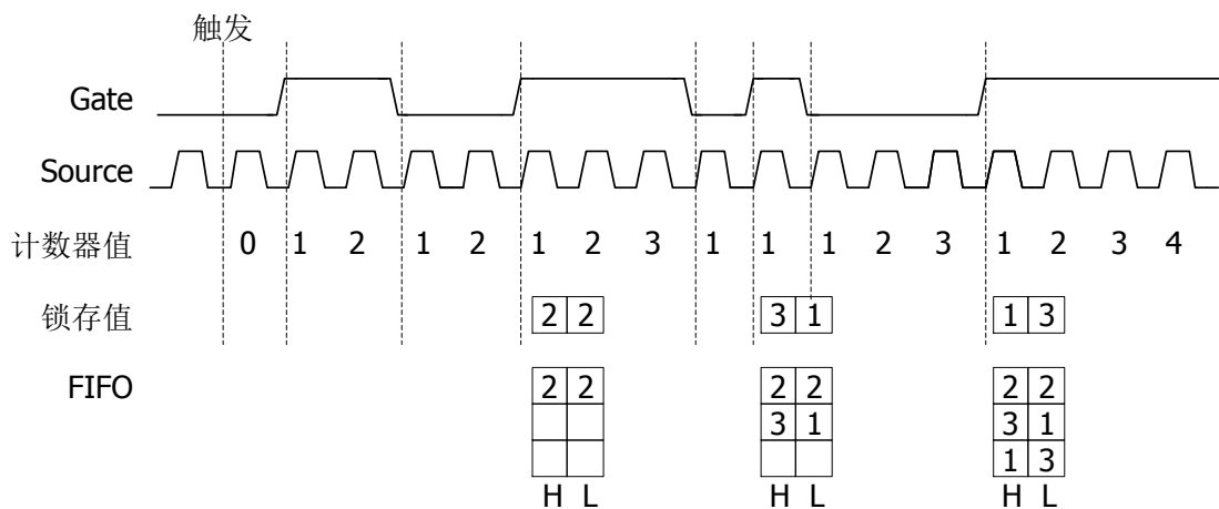
图 7.9 隐式缓冲脉宽采集示例
