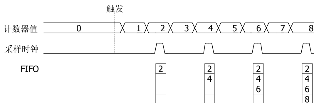
图 7.24 采样时钟定时连续采集示例
