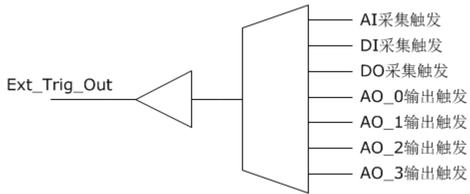
图 8.4、外触发输出电路示意图
