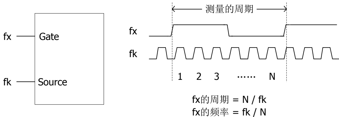
图 7.13 频率（周期）测量原理
