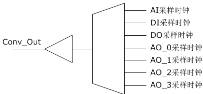
图 8.2、采样时钟输出电路示意图
