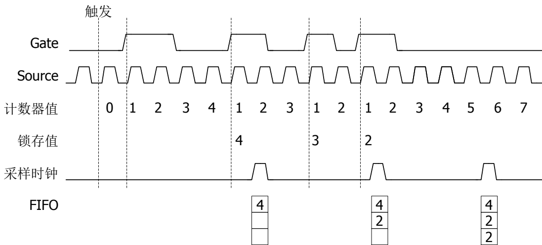
图 7.15 采样时钟定时连续采集示例
