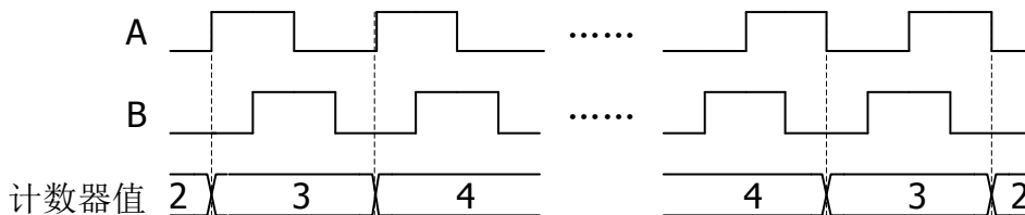
图 7.17 正交编码器 X1 编码计数方式
